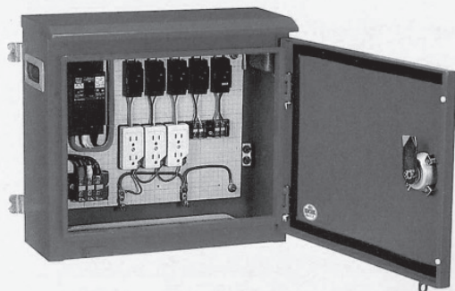
電灯分電盤 S50-5型
