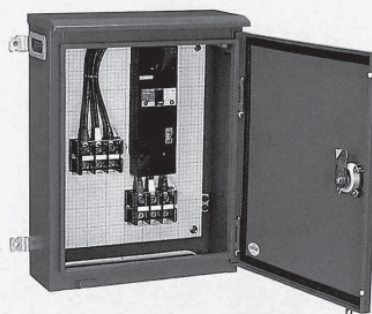
動力主幹盤 P100-1型
