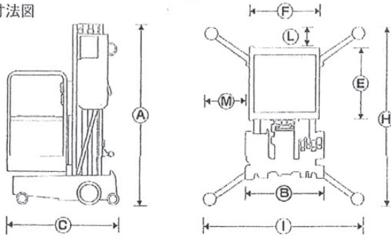
■車両寸法図
