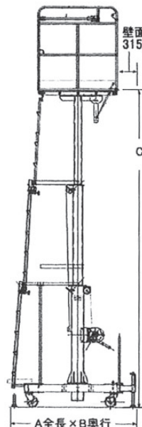
■側面伸長図
