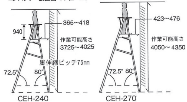
コンスタワー設置図 (単位: mm)
